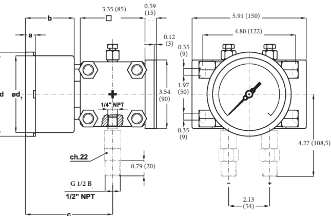
Нижний монтаж (Код A для монтажа) , с задним фланцем (Опциональный код C): DS 4", 6" (100-150мм)
