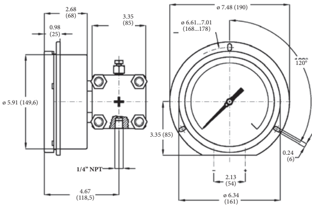
Нижний монтаж (Код A для монтажа) , с передним фланцем (Опциональный код E): DS 6" (150мм)
