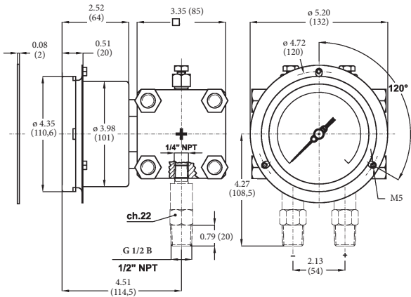
Нижний монтаж (Код A для монтажа) , с передним фланцем (Опциональный код F): DS 4" (100мм)
