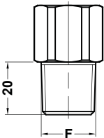
43M - 1/2-18 NPT
